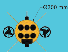
偵搜型 Module A (偵搜繫流雷 For Mooring Mine)
